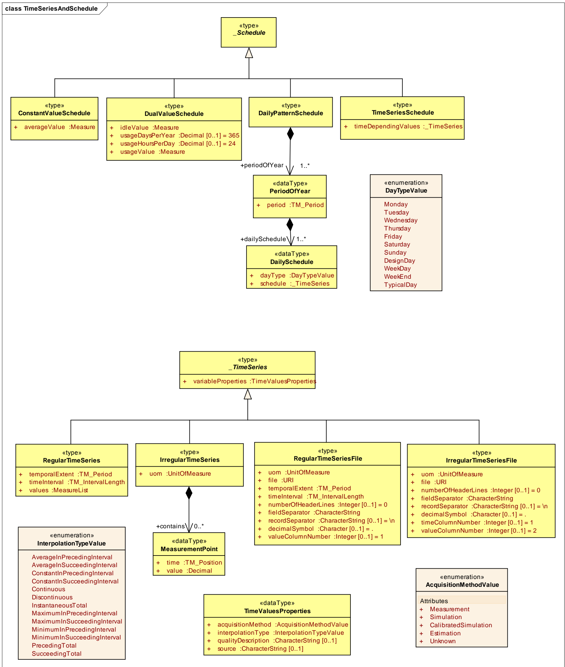
Diagram: TimeSeriesAndSchedule
