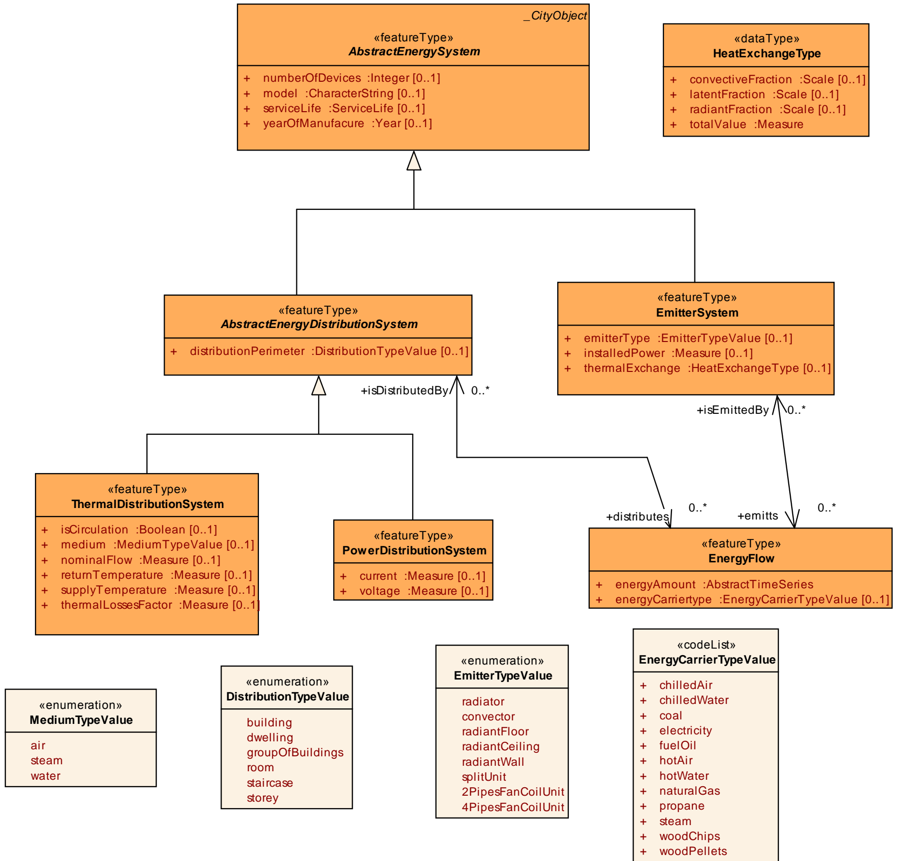
Diagram: EnergyDistributionEmissionSystem
